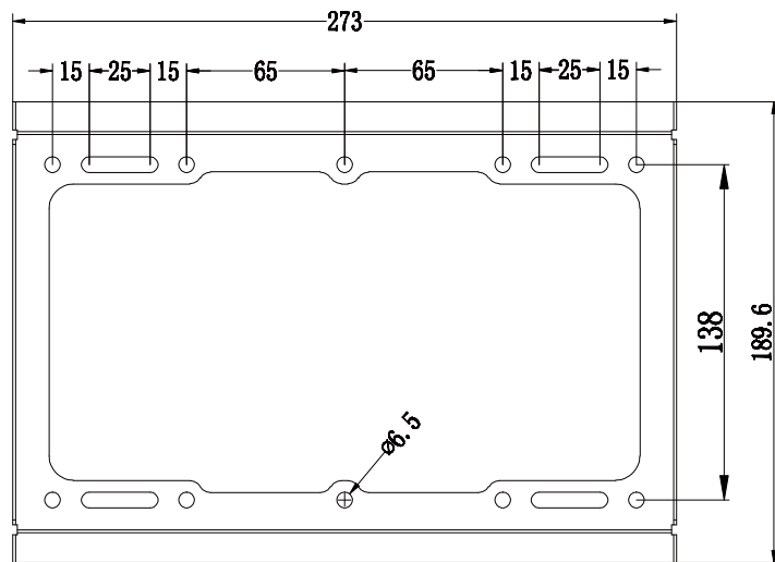
【正面図（壁側）】
