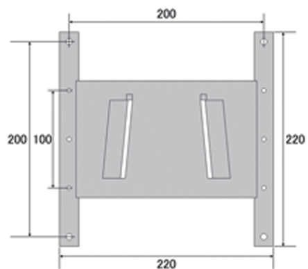
【テレビ側取付金具寸法】
