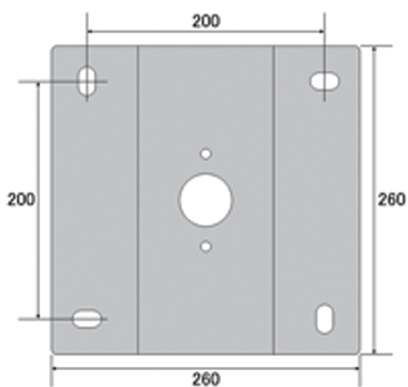
【天井ベース寸法】
